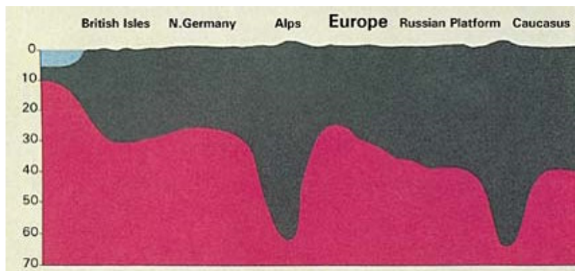
Figur 8: Skematisk tværsnit. Bjergene, som pløkker, har dybe rødder indlejret i jorden. ( Anatomy of the Earth , Cailleux, s. 220).
