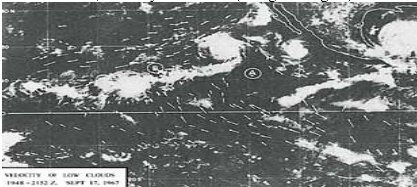
Figur 17: Satellitbillede der viser skyer, som bevæger sig mod konvergensområderne B, C og D. Pilene viser vindretningen. ( The Use of Satellite Pictures in Weather Analysis and Forecasting , Anderson et al., s. 188).
