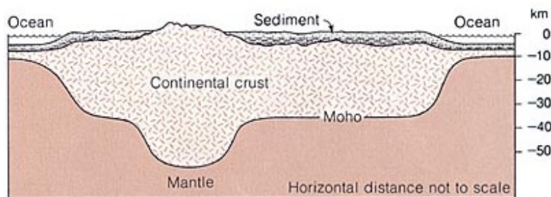
Figur 7: Bjerge har dybe rødder under jordoverfladen. ( Earth , Press og Siever, s. 413).
