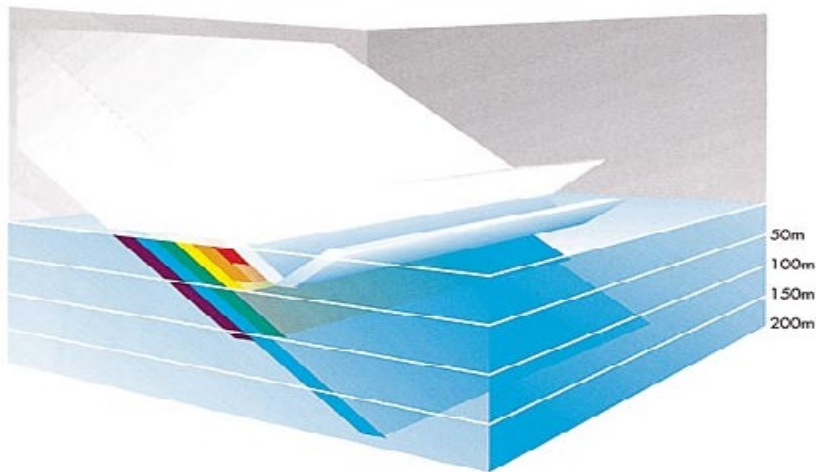
Figur 15: Mellem 3 og 30 procent af sollyset reflekteres ved vandoverfladen. Så absorberes næsten alle syv farver i spektret en efter en i de første 200 m, undtagen det blå lys. ( Oceans , Elder og Pernetta, s.27).
