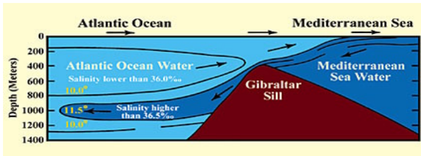
Figur 13: Middelhavsvandet idet det kommer ind i Atlanterhavet over Gibraltartærsklen med dets eget varme, saltholdige og mindre tætte egenskaber pga. grænsen, der skiller dem. Temperaturerne er i celcius. ( Marine Geology , Kuenen, s. 43, med mindre ændringer).
