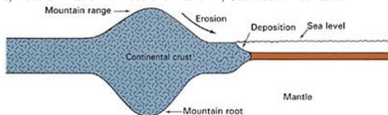
Figur 9: En anden illustration der viser, at bjerge har form som en pløk, pga. deres dybe rødder. ( Earth Science , Tarbuck og Lutgens, s. 158.)
