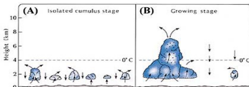
Figur 19: (A) Isolerede små stumper af skyer (cumulusskyer). (B) Når de små skyer samler sig, tiltager opdriften i den større sky, så skyen stakkes op. De små prikker er vanddråber. ( The Atmosphere , Anthes et al., s 269)
