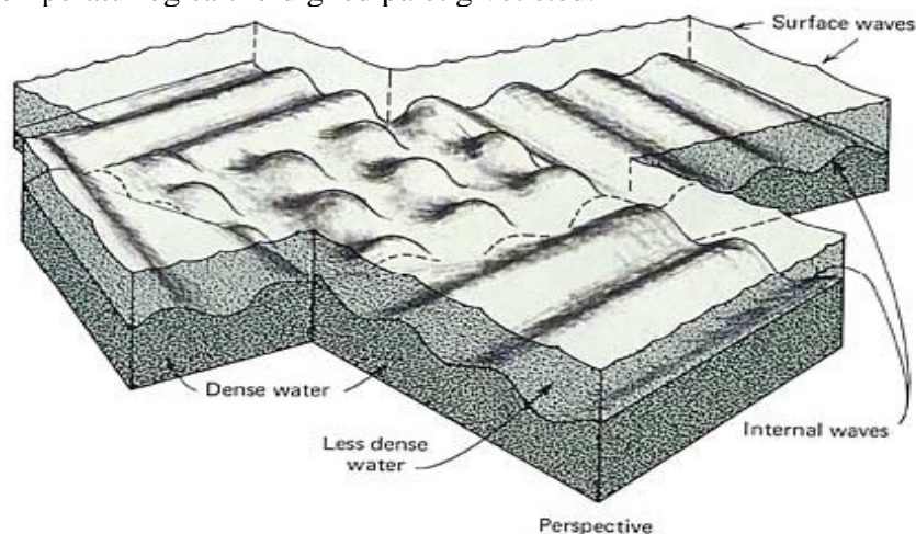
Figur 16: Indre bølger ved grænsen mellem to lag vand af forskellig tæthedsgrad. Det ene er tæt (det dybe), det andet er mindre tæt (det øverste) ( Oceanography , Gross, s. 204).
