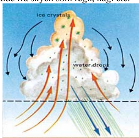
Figur 20: En Cumulonimbus sky. Efter skyen er stakket op, kommer regnen ud af den. ( Weather and Climate , Bodin, s. 123) (Tekst i figur 20: Iskrystaller, vanddråber).
