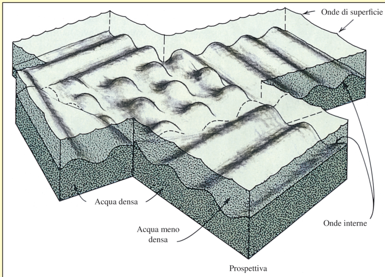
Figura 16: Onde interne sull' interfaccia tra che si trova tra due strati d'acqua di diversa densità. Una è densa (la più profonda), l'altra è meno densa (la più superficiale). ( Oceanography (Oceanografia), Gross, p. 204.)
