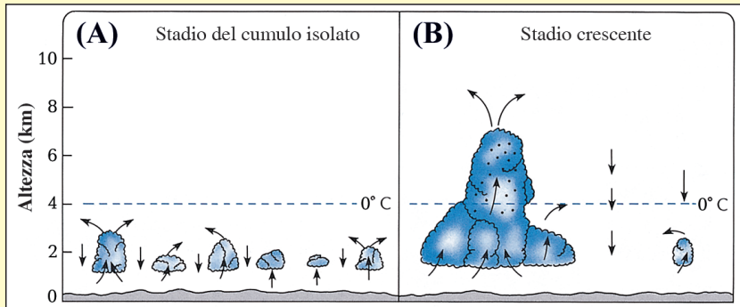
Figura 19: (A) Piccole nubi isolate (nubi cumulo). (B) Quando le piccole nubi si uniscono, le correnti ascensionali all'interno della grossa nube aumentano, cos  la nuvola si ingrandisce. Le gocce di pioggia sono indicate con \cdot . ( The Atmosphere (Atmosfera), Anthes e altri, p. 269.)
